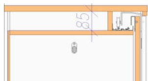
Detail oben
